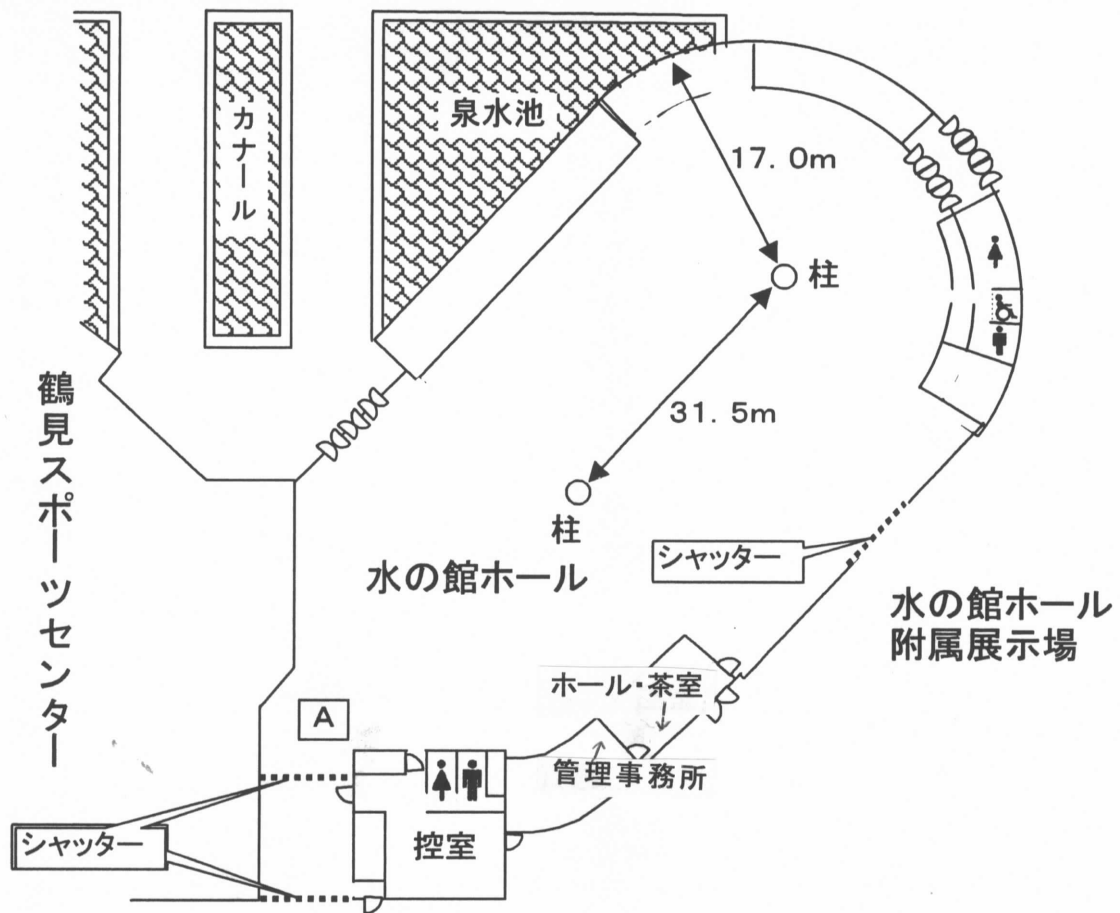
水の館ホール平面図
